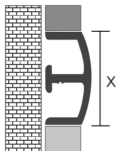
Dekorcsík, alumínium
