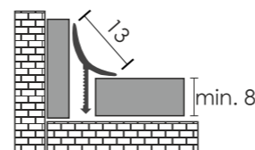
Beépíthető belső sarokélvédő, (lábatlan), alumínium
