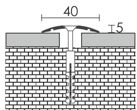
Furatos "lencse" burkolatváltó, alumínium
