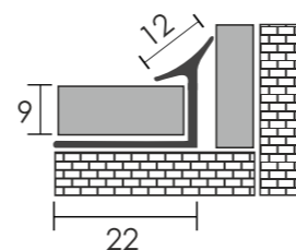
Beépíthető belső sarokélvédő, (lábás), alumínium
