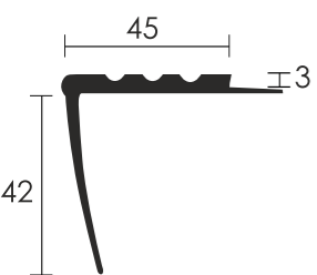
Lépcsőélvédő, lágy PVC
