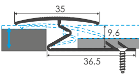
Roppantós burkolatváltó, alumínium
