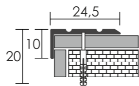
Furatos lépcsőélvédő, alumínium
