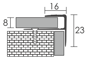
Lépcsőélvédő laminált padlóhoz, alumínium
