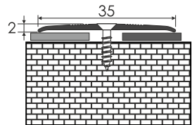
Furatos burkolatváltó, alumínium
