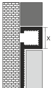
Dekorációs élvédő, alumínium
