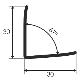
Lépcsőszőnyeg profil, PVC
