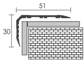
Utólagos lépcsőélvédő alapsín, alumínium Öntapadós csúszásgátló betét
