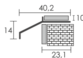
Vízvető teraszprofil, alumínium
