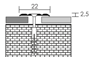
Furatos burkolatváltó, alumínium
