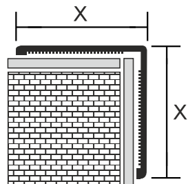
Sarokélvédő, alumínium
