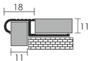
Íves lépcsőélvédő, alumínium
