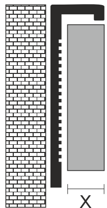
Hajlítható élvédő, alumínium
